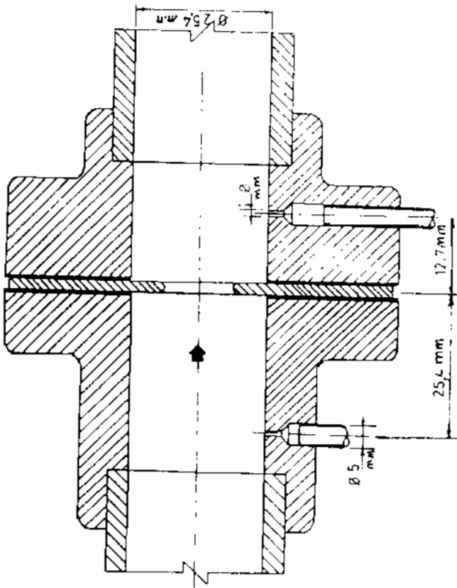
Fig( 2 ) Driftice meter
